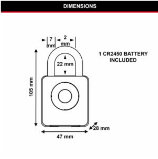
4400EUREC_DIMENSIONS
